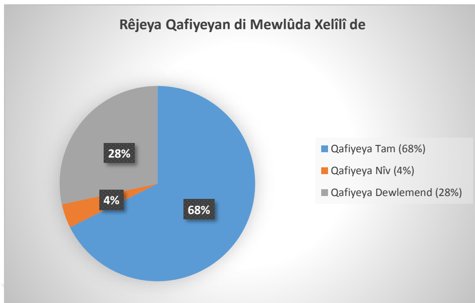
Grafîk 2: Li gorî hejmara beytan rêjeya qafiyeyan di mewlûda Xelîlî de.
