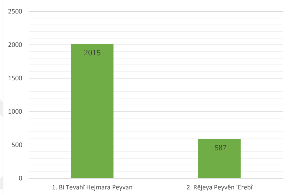
Grafîk 1: Bi tevahî hejmara peyvan û hejmara peyvên 'Erebî.
