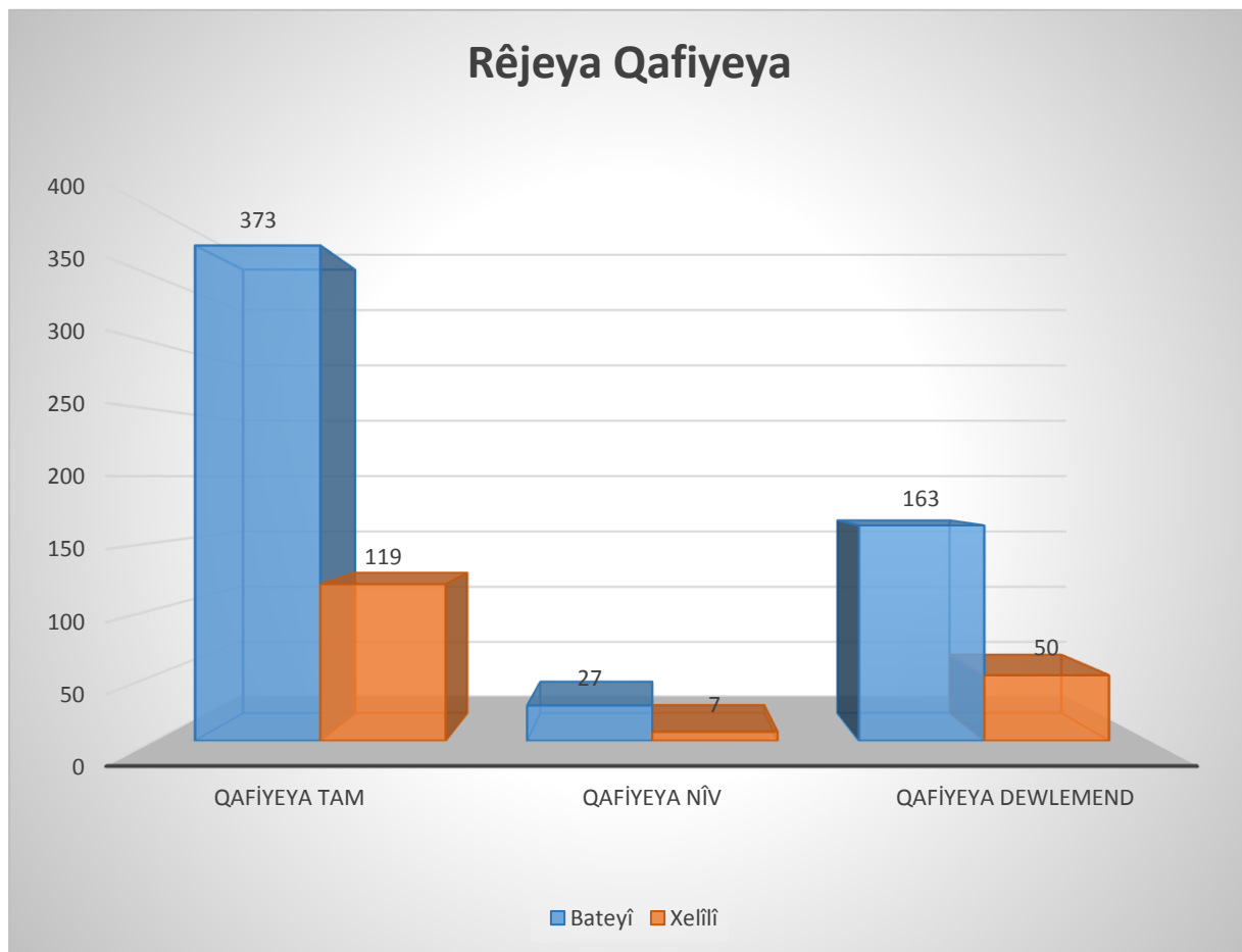
Grafîk 4: Li gorî hejmara beytan rêjeya qafiyeyan di her du mewlûdan de
