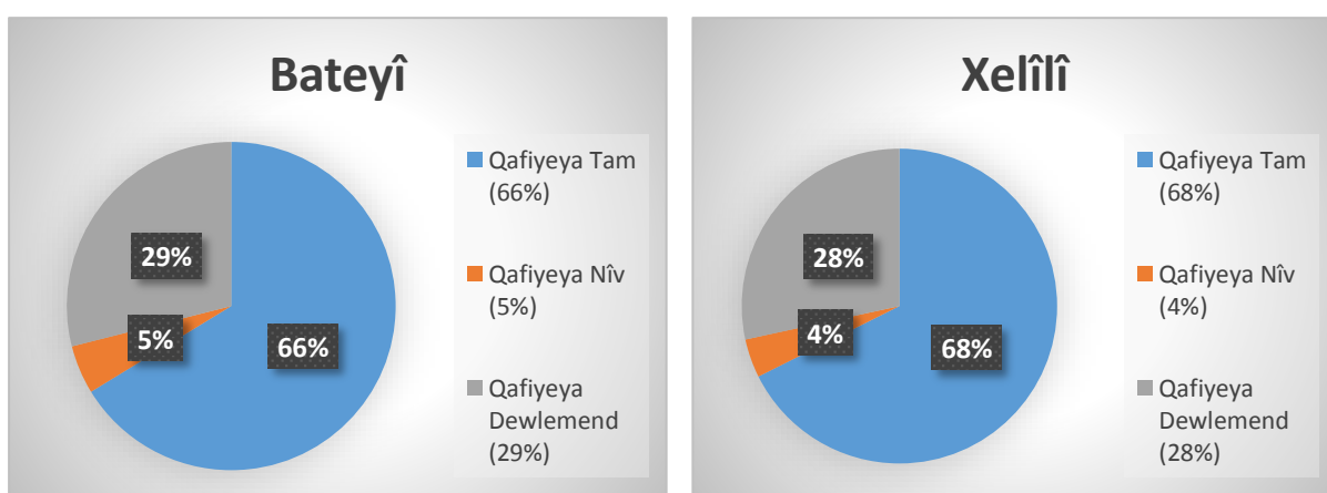
Grafîk 5: Berawirdkirina hejmara qafiyeyan di her du mewlûdan de
