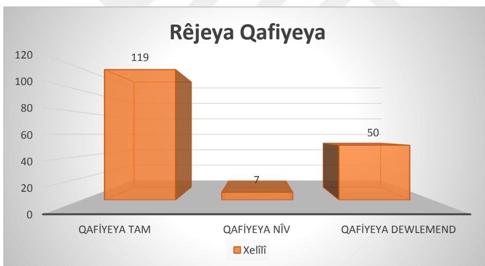
Grafîk 3: Hejmara cureyên qafiyeyan di mewlûda Xelîlî de.
